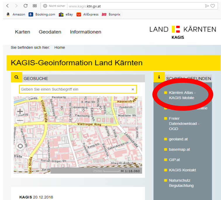
Abbildung 1: KAGIS Homepage
